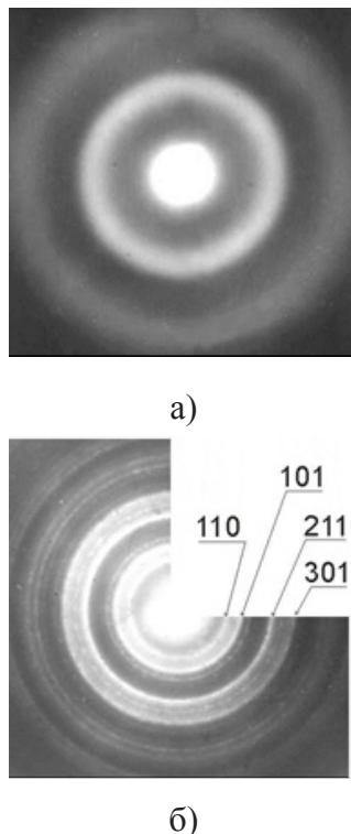
Рисунок 4. Дифракция электронов для пленочных образцов диоксида олова с толщиной меньшей (а) и большей (б) h_{\text{кр}} .
