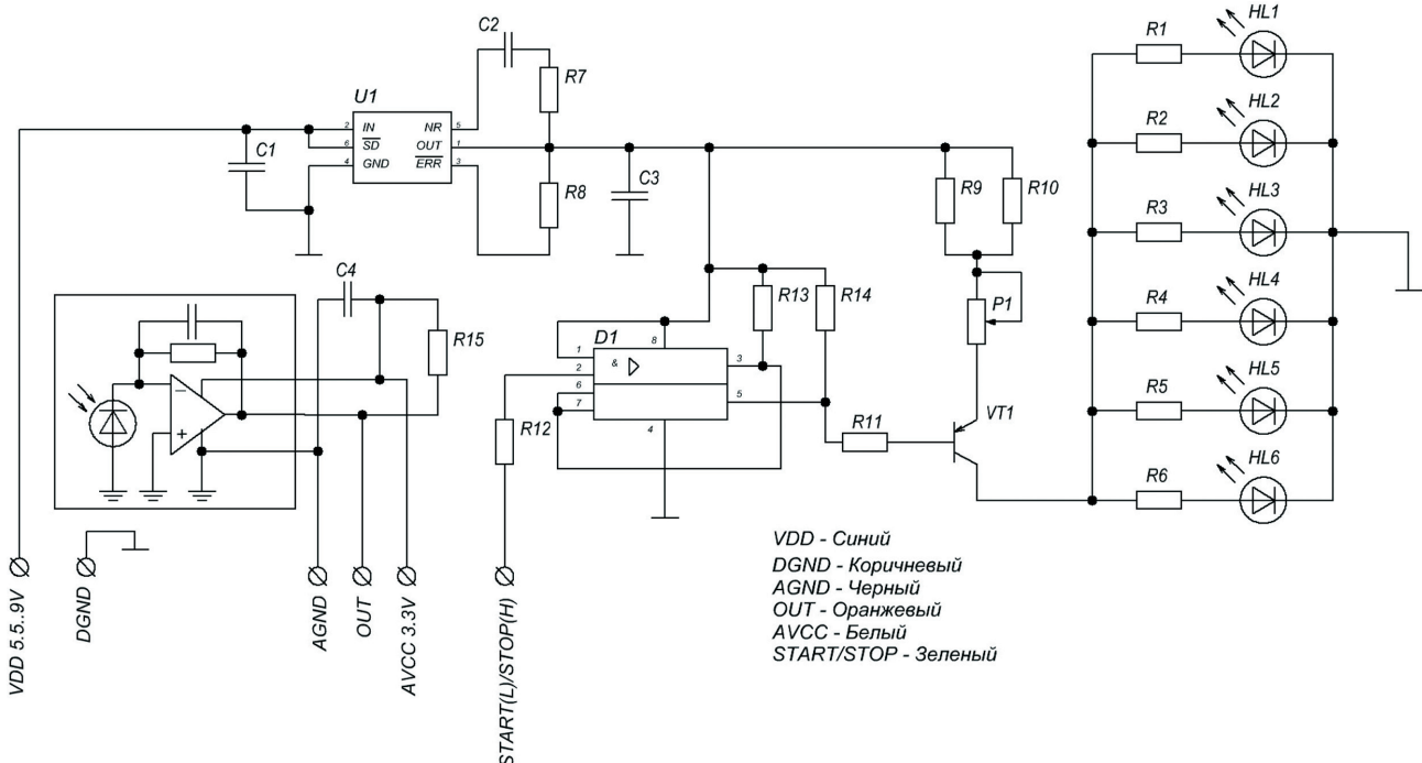
Рис.1. Принципова електрична схема сенсора.
