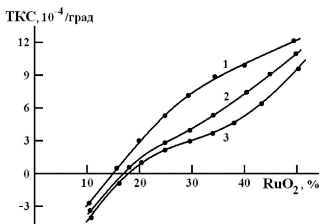
Рис. 3. Зависимость ТКС от концентрации \text{RuO}_2 . Время ультразвуковой обработки, мин.: 1 – 0, 2 – 90, 3 – 180. Температура вжигания 870^\circ\text{C}
