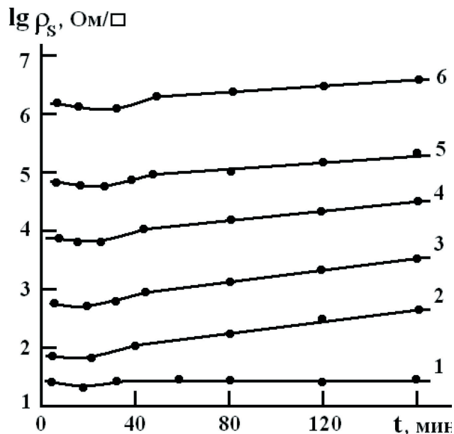
Рис. 4. Зависимость удельного поверхностного сопротивления \rho_s от времени ультразвуковой обработки. Концентрация \text{RuO}_2 , мас. %: 1 – 10, 2 – 15, 3 – 20, 4 – 30, 5 – 40, 6 – 50
