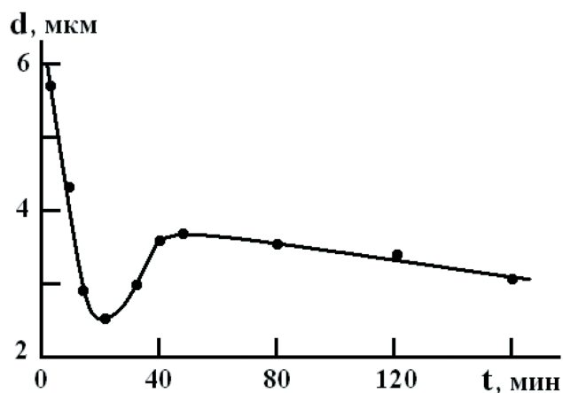
Рис. 1. Зависимость средних размеров агломератов частиц \text{RuO}_2 от времени ультразвуковой обработки
