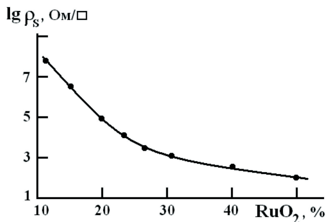
Рис. 2. Зависимость удельного поверхностного сопротивления \rho_s структур “ \text{RuO}_2 – стекло” от концентрации \text{RuO}_2 (без ультразвуковой обработки). Температура вжигания 870 °С
