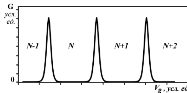
Рис. 6. Кулоновские осцилляции
