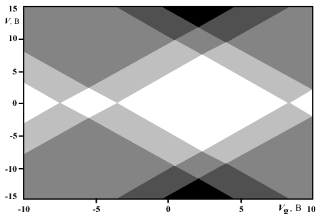
Рис. 10. Диаграмма зарядовой стабильности, иначе, диаграмма кулоновской блокады, полевого транзистора на молекуле бензола, вычисленная из первых принципов. Диаграмма показывает число заряженных состояний молекулы в канале туннелирования в зависимости от значений V и V_g : в белых полях заряженных состояний нет («кулоновская блокада»), в остальных полях число заряженных состояний изменяется от 1 до 4, возрастающая с плотностью закрашки полей. Из-за некоторого сходства многоугольников с гранями алмаза подобные графики в англоязычной литературе принято называть кулоновскими алмазами (Coulomb diamonds)
