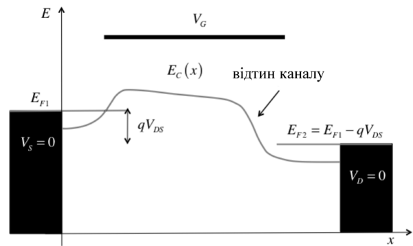
Рис. 21. Схематичний хід E_C(x) для транзистора з довгим каналом провідності при високих значеннях напруги як на затворі, так і на стоку. У цьому випадку низьке зовнішнє електричне поле «покриває» значну частину каналу провідності й область відтину каналу невелика. Додаткове збільшення напруги на стоку дещо збільшує область відтину, довжина якої, однак, охоплюватиме лише невелику частину довгого каналу провідності.
