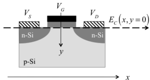
Рис. 12. Переріз n -MOSFET і система координат, використовувана для графічного зображення енергії в залежності від координати точки при рухові від витіку вздовж каналу провідності до стоку. Вісь z направлено за рисунок вздовж ширини каналу провідності W .
