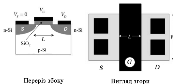
Рис. 3. n -канальний Si MOSFET: переріз (вигляд збоку) і вигляд згори. Схематично зображено контакти витоку та стоку (чорні квадрати) та затвору (чорний прямокутник).
