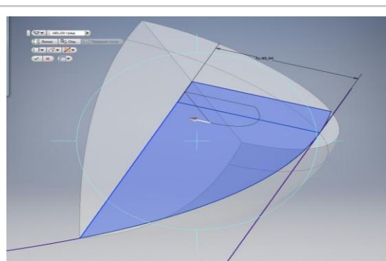
На відміну від параболоїда обертання, тороїдально-параболічне дзеркало будується обертанням параболи навколо вісі паралельній вісі x на відстань F \cdot k , де k - варійований параметр
